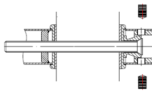
Wood or Metal Door Mount
