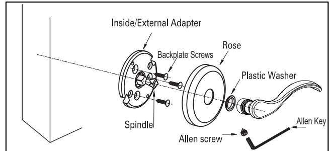
Exploded View Dummy Lockset Despiece de Cerradura Dummy Éclaté des Serrures Rossace
